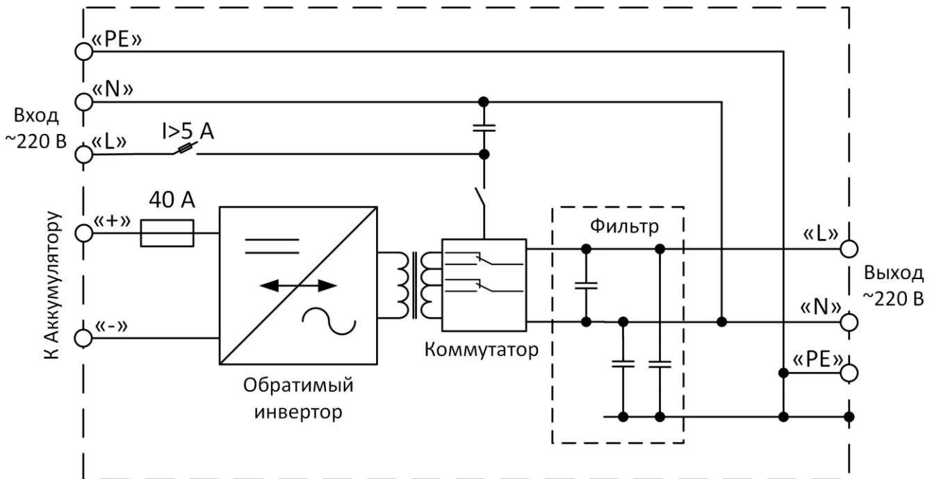
Рисунок 4. Блок-схема ИБП КУЛОН в режиме работы от батареи
