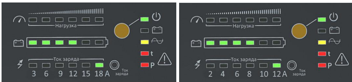
Рисунок 2. Зовнішній вигляд панелі керування ДБЖ на 300 та 180ВА
