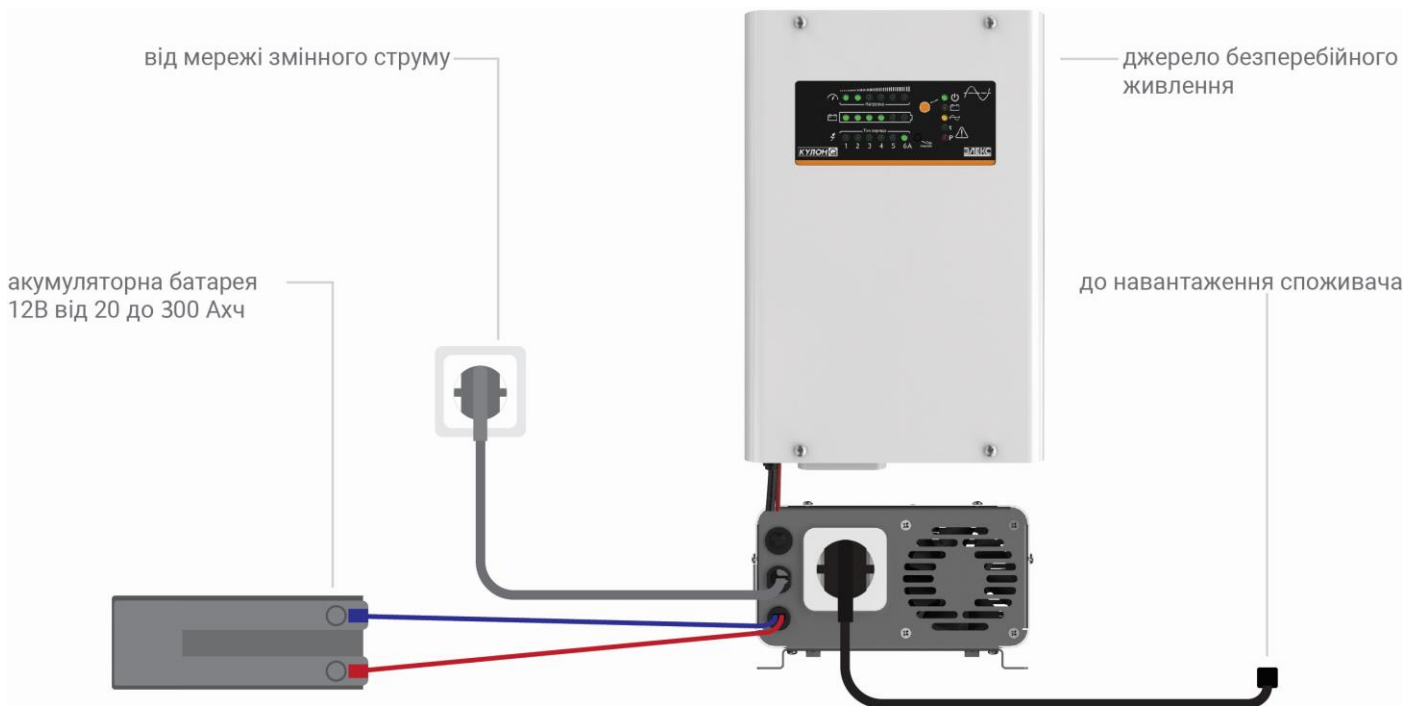
Рисунок 6. Схема підключення ДБЖ до силової мережі
