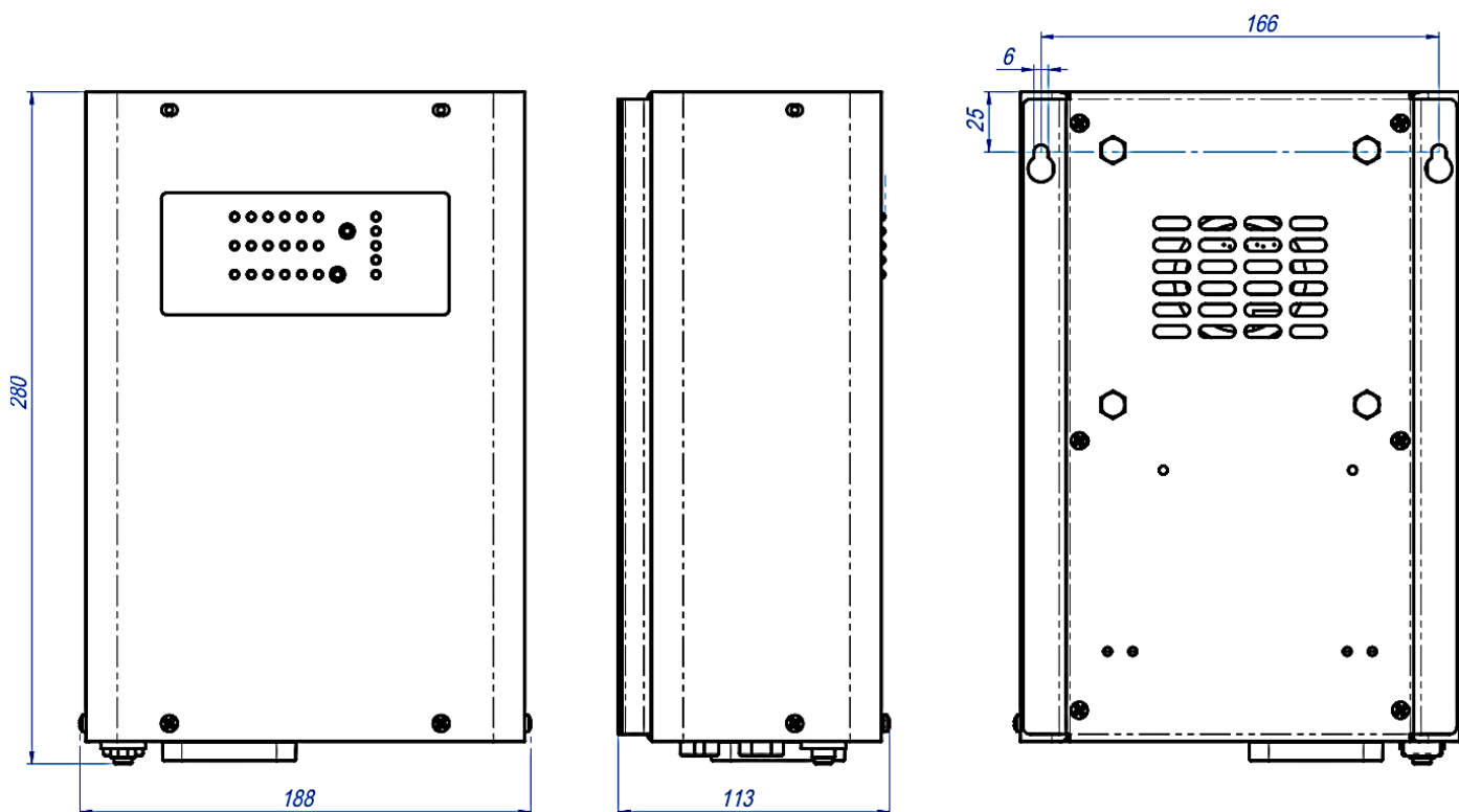
Рисунок 5. Установочные и посадочные размеры ИБП
