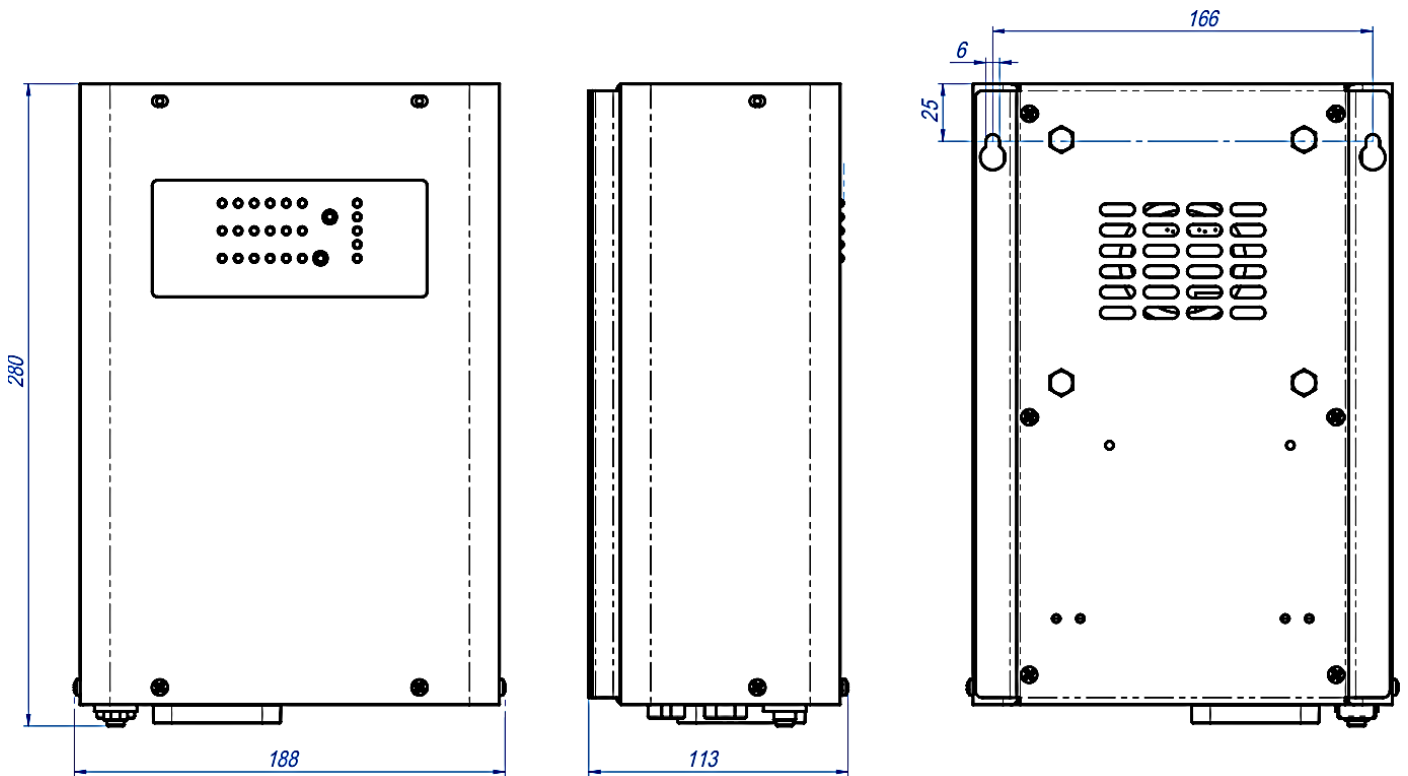
Рисунок 5. Установчі та посадочні розміри ДБЖ
