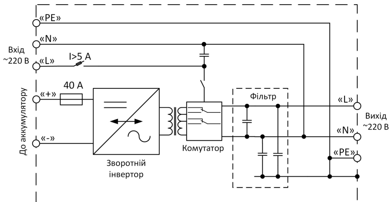
Рисунок 4. Блок-схема ДБЖ КУЛОН при роботі від батареї
